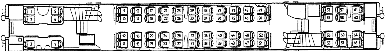
Ed Doppelstockwagen (I) mit Mittelgang/Voiture Ed (I) à deux niveaux à couloir central/Ed double-deck coach (I) with central corridor
