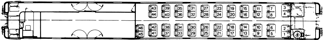
Ein Wagen mit Mittelgang/Voiture Ein à couloir central/Ein coach with central corridor -2. Klasse/2 e classe
