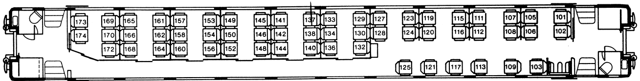
Cx Wagen (I) mit Seiten- und Mittelgang/Voiture Cx (I) à couloir latéral et central/Cx coach (I) with lateral and central corridors 1. Klasse/1 e classe
