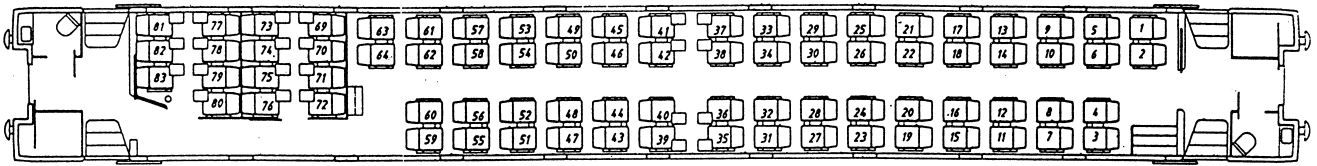
Ex Wagen (I) mit Mittelgang/Voiture Ex (I) à couloir central/Ex coach (I) with central corridor -2. Klasse/2 e classe
